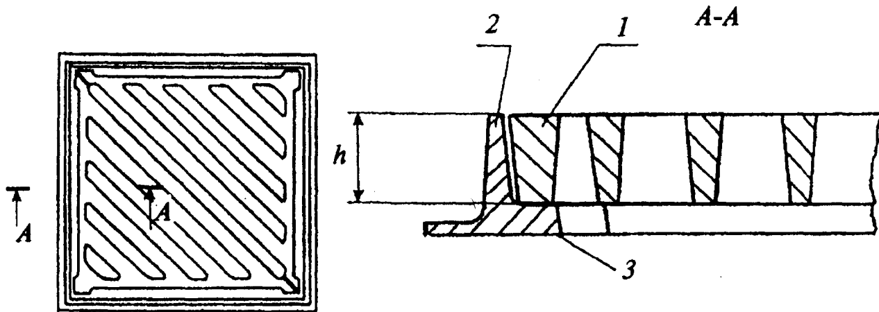
1 — крышка; 2 — корпус; 3 — опорная поверхность корпуса Рисунок Б.1 — Дождеприемник ливнесточного колодца
